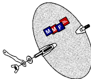
Damper Disc ----- Page 40A
